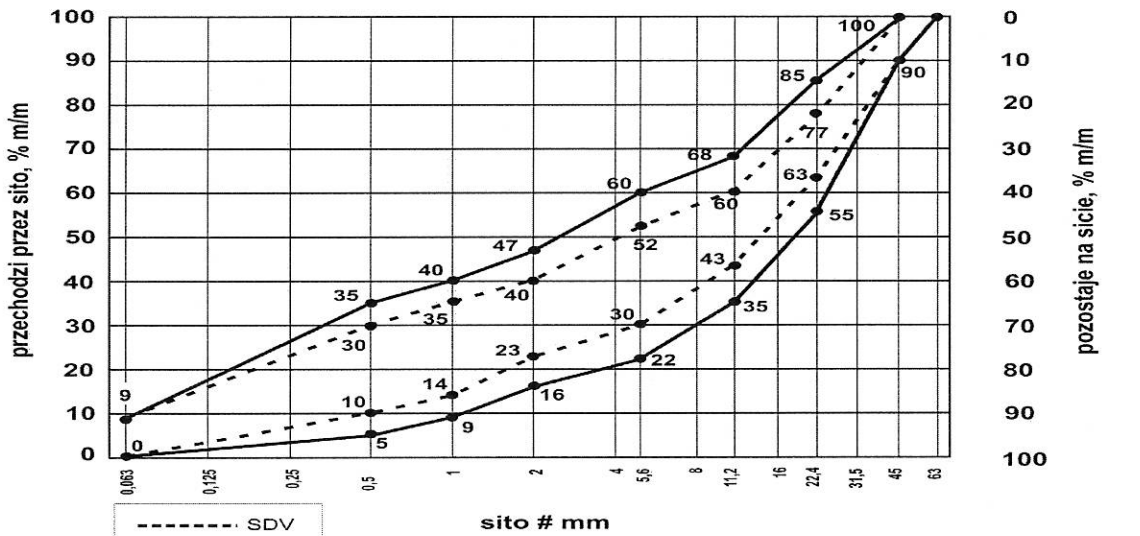
Rys. 12. Uziarnienie mieszanki niezwiązanej 0/45 dla podbudowy zasadniczej
